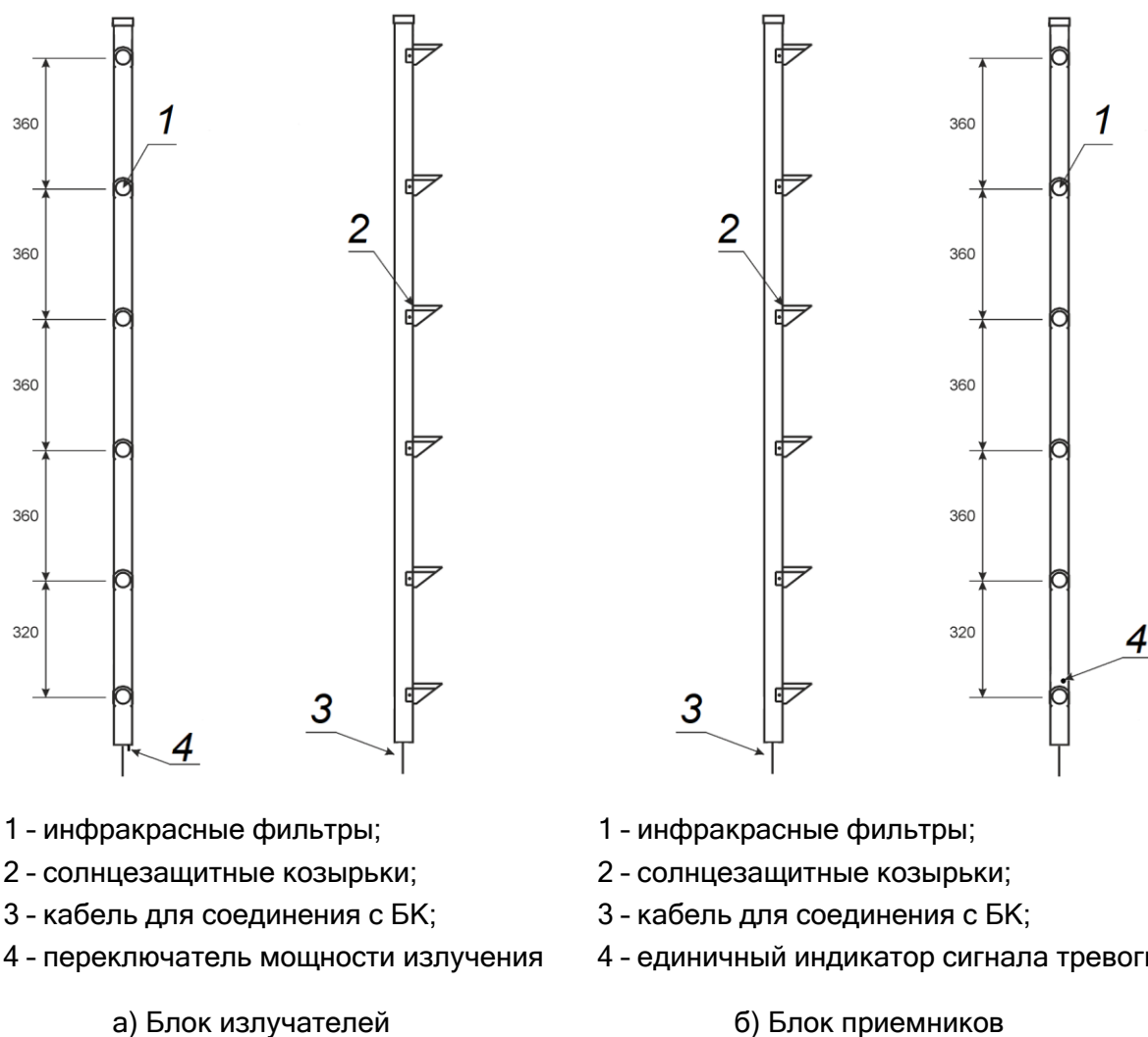
Рисунок 1.2 - Общий вид БИ и БП
